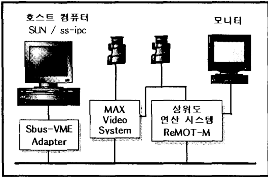
그림 8. 실험에 사용한 하드웨어의 구성
