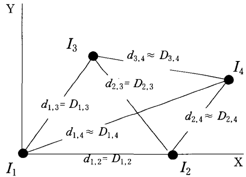
그림 3. 상위도공간에서 4매의 영상( I_1 \sim I_4 )을 배치시킨 모습(본문참조). “ \approx ”기호는 두 영상간의 상위도 D_{i,j} 와 공간상의 거리 d_{i,j} 가 근사적으로 일치함을 의미한다.
