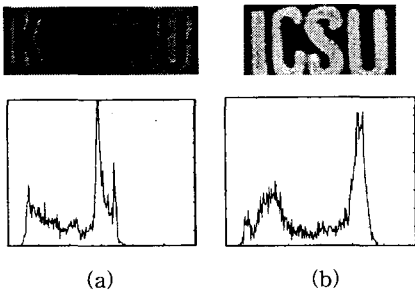
그림 11. (a) 패널이 있는 경우와 (b) 문자의 화소가 배경의 화소보다 많은 경우의 영상과 히스토그램.
