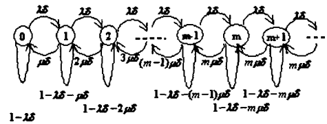
<그림 7> M/M/m Markov 프로세스
