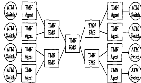
<그림 4> ETRI ATM교환기 TMN시스템
