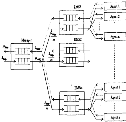
<그림 5> TMN EMS 성능 평가 모델
