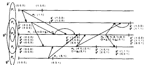
그림 3. 레벨 2 수신자 선택 알고리즘의 예 다음은 수신자 선택 알고리즘을 기술하였으며, 그림 3은 제안된 알고리즘의 예를 보여준다.
