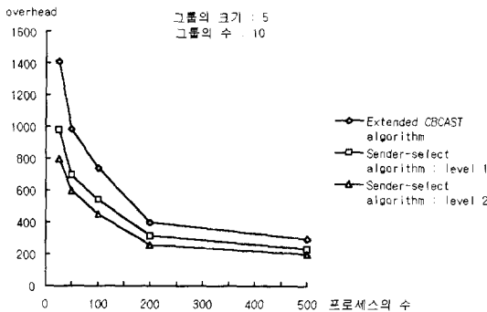
그림 5. 프로세스 수의 변화에 따른 각 알고리즘의 오버헤드
