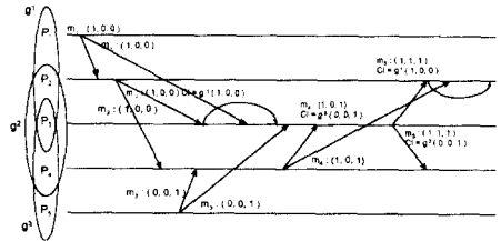
그림 2. 송신자 선택 알고리즘의 예
