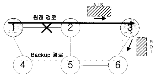
그림 2.2 Backup VP를 이용한 복구 (Restoration using Backup VP)
