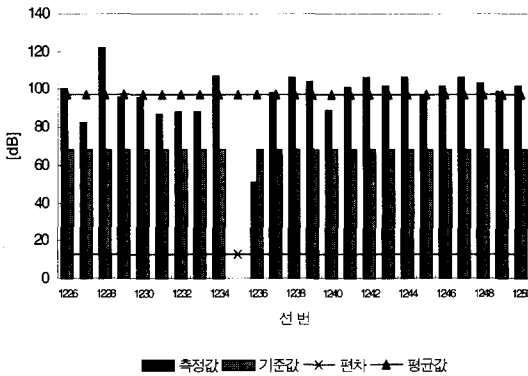
(a) C-44 1235 선번의 field data
