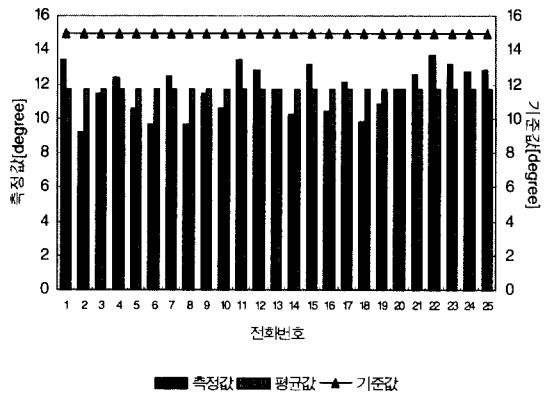
(d) 위상지터의 통계처리
