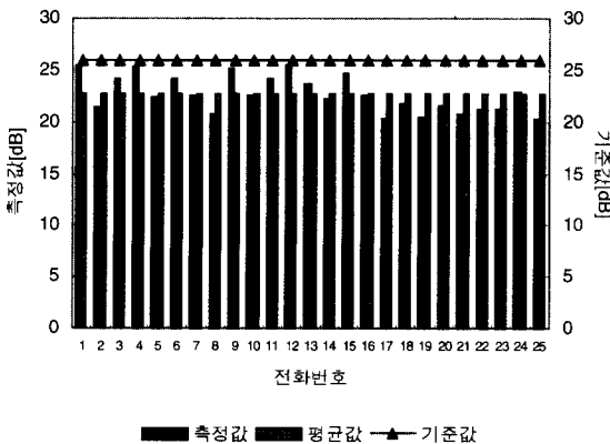
(a) 전송손실의 통계처리
