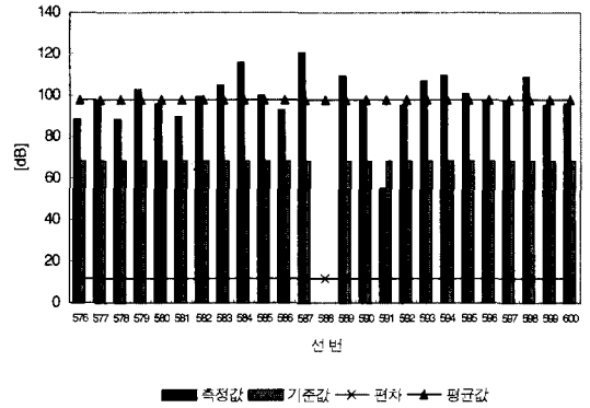
(c) C-45 588 선번의 field data
