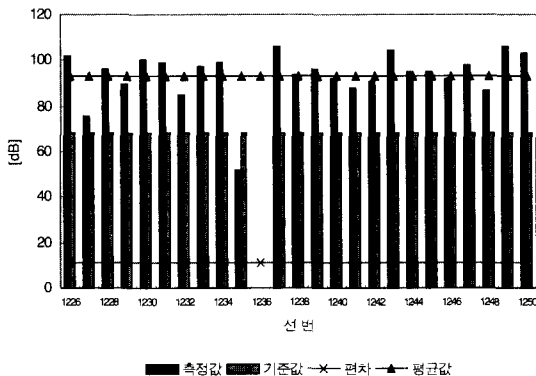
(b) C-44 1236 선번의 field data
