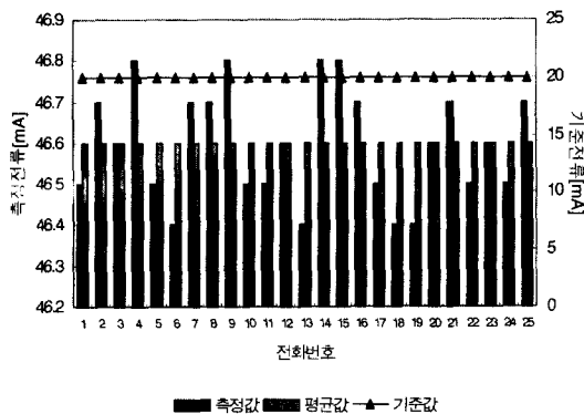
(b) 공급전류의 통계처리
