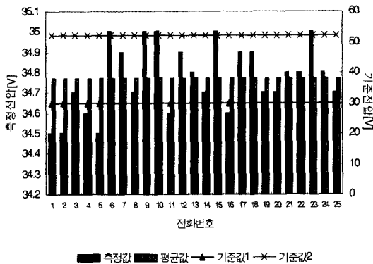
(a) 공급전압의 통계처리
