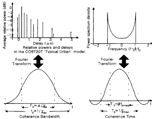
그림 1. 무선통신 채널특성
