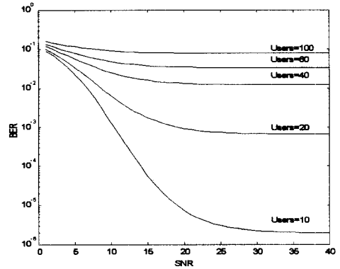
그림 6. 완벽한 채널추정 시 SNR에 따른 BER 성능
