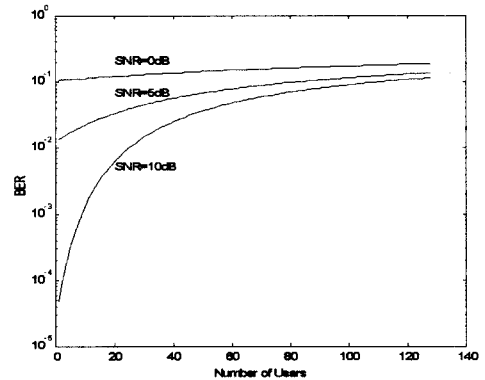
그림 7. 완벽한 채널추정시 사용자 수에 따른 BER 성능
