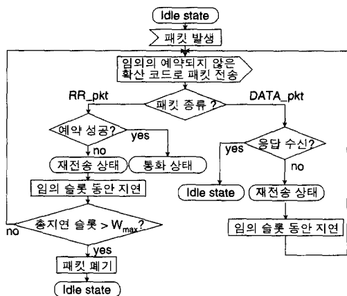
그림 3. RRA_CDMA 프로토콜의 동작
