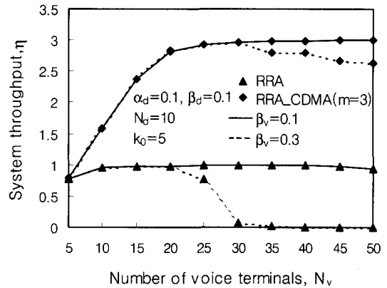
그림 6. 시스템 처리율
