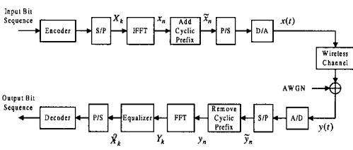
그림 1. 기저대역 OFDM 시스템의 블록도
