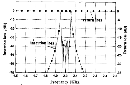
그림 12. 1.5~2.5 GHz 대역에서의 시뮬레이션 결과
