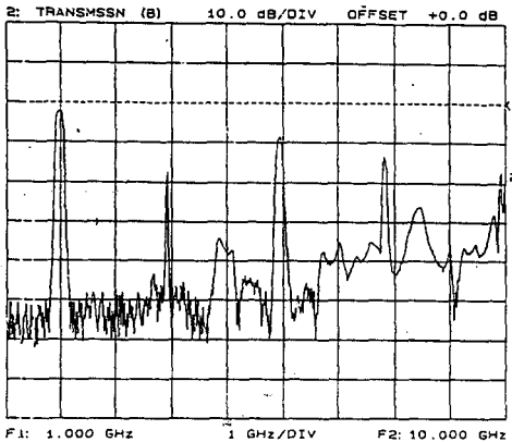
그림 18. Hairpin Line 여파기의 1~10 GHz 대역에서의 감쇄 특성
