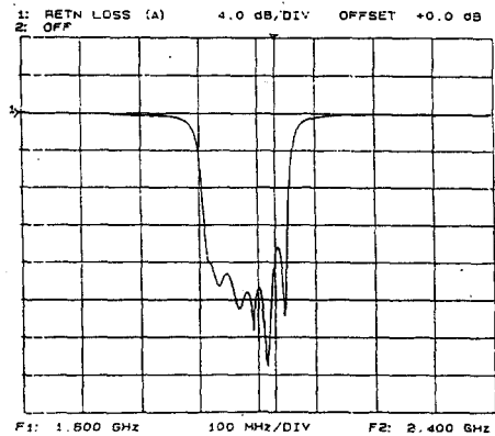
그림 17. Hairpin Line 여파기의 반사 손실 특성
