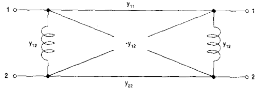
그림 2. 2선 결합 전송 선로의 그래프 표현
