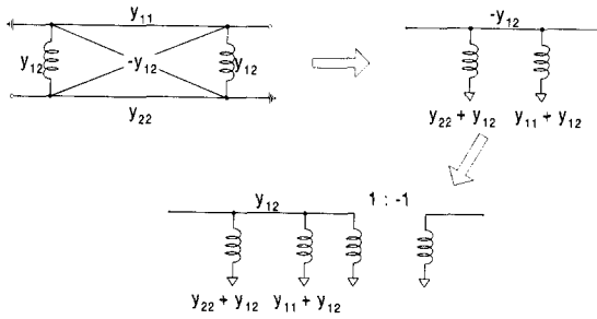
그림 5. 그림 3의 (b)에 대한 등가회로의 유도
