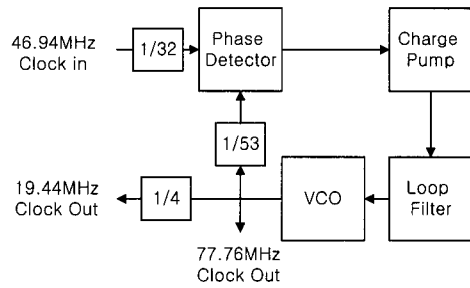
그림 5. 가입자 클럭 발생용 PLL 회로의 블록도
