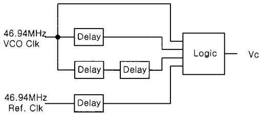
그림 3. 위상비교기 회로 블록도
