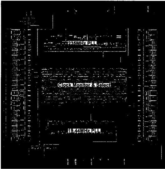
그림 9. 설계된 칩의 layout.
