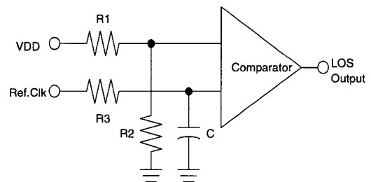
그림 6. LOS 회로도
