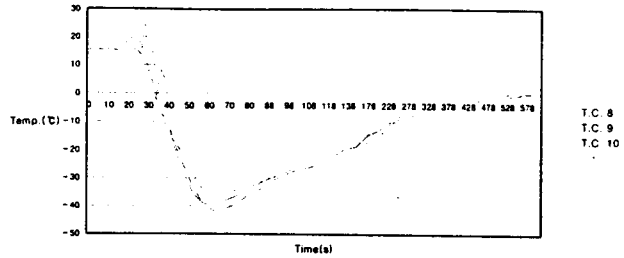
그림 11. Lower Layer Temp. profile of Experiment No. 3
