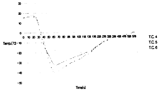
그림 10. Upper and Middle Layer Temp. profile of Experiment No. 3
