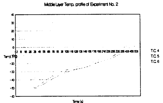
그림 7. Middle Layer Temp. profile of Experiment No. 2
