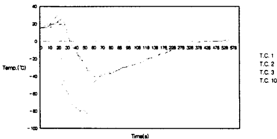
그림 9. Upper Layer Temp. profile of Experiment No. 3
