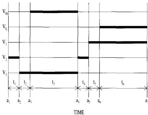
그림 5 3중 버퍼 맥동관 냉동기의밸브 타이밍 Fig. 5. Valve timing of three buffer pulse tube refrigerator
