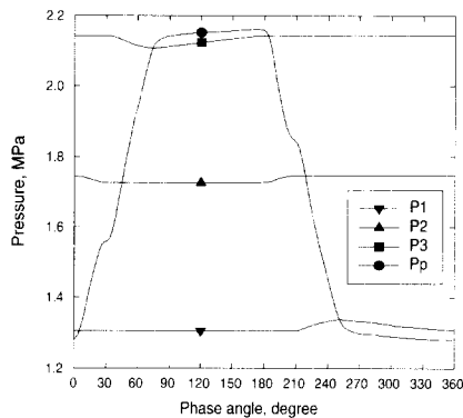
그림 3 3중 버퍼 맥동관 냉동기의 압력변화 Fig. 3. Typical pressure wave of three buffer pulse tube refrigerator
