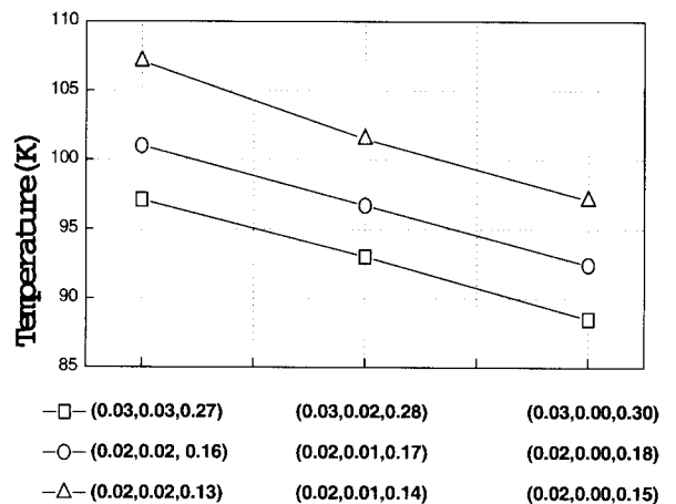
그림 9 작동주파수와 밸브 타이밍에 따른 최저도달온도 변화
