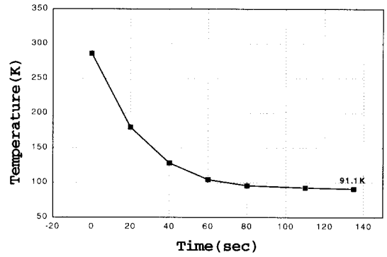
그림 7 3중 버퍼 맥동관 냉동기의 냉각 특성
