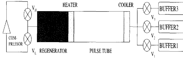
그림 4 3중 버퍼 맥동관 냉동기의 개략도 Fig. 4. Three buffer pulse tube refrigerator
