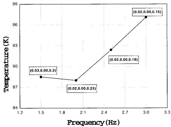
그림 10 작동주파수에 따른 최저도달온도 변화 Fig. 10. No load temperature as a function of operating frequency
