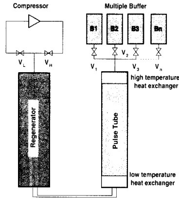
그림 1 n 버퍼를 가진 MBPTR의 개략도 Fig. 1. Schematic diagram of MBPTR
