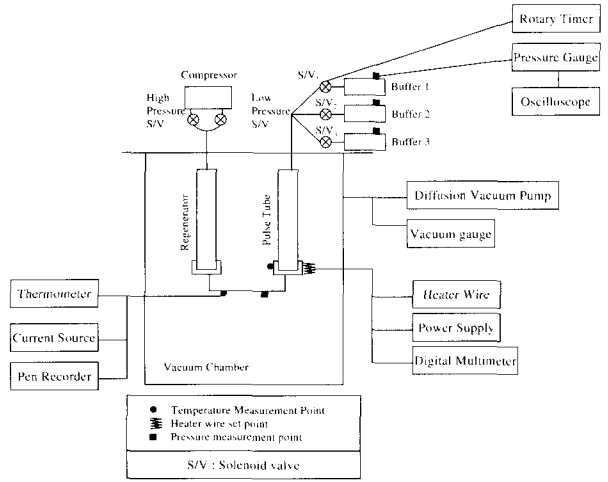
그림 6 3중 버퍼 맥동관 냉동기의 실험장치 개략도 Fig. 6. Experimental apparatus of three buffer pulse tube refrigerator
