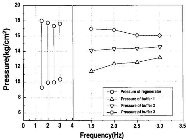
그림 11 작동주파수에 따른 압력변화 Fig. 11. Pressure variation as a function of operating frequency
