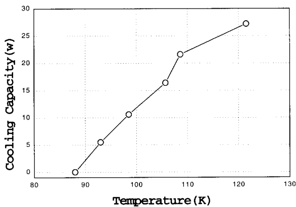
그림 12 3중 맥동관 냉동기의 냉동능력 Fig. 12. Load characteristics of three buffer pulse tube refrigerator
