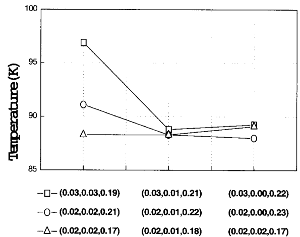
그림 8 반주기 시간비율과 밸브 타이밍에 따른 최저도달온도 변화
