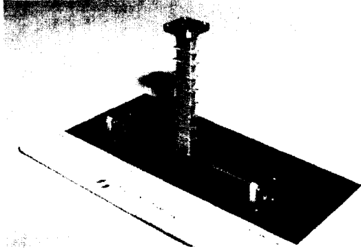
그림 10. 제작된 Ka-밴드 위성중계기용 다이플렉서 Fig. 10. Fabricated diplexer for Ka-band transponder.
