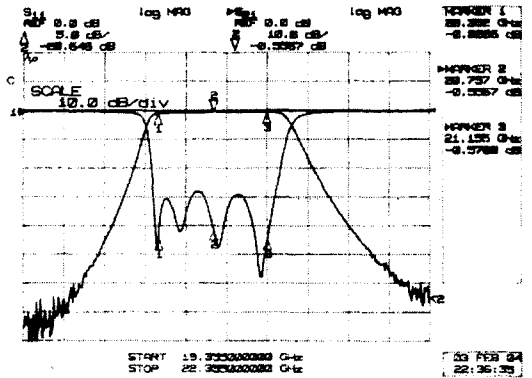
그림 12. 수신 필터의 전달특성 Fig. 12. Transmission characteristics of Rx filter.
