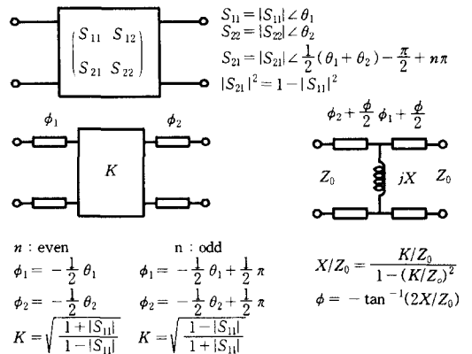
그림 6. 산란행렬에 의한 임피던스 인버터의 크기 및 위상 계산
