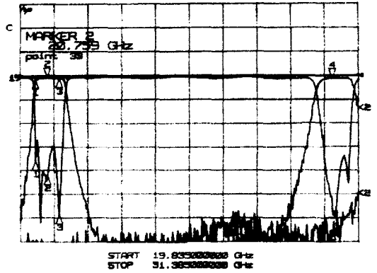
그림 11. 송·수신 필터의 전달특성 Fig. 11. Transmission characteristics of Rx and Tx.
