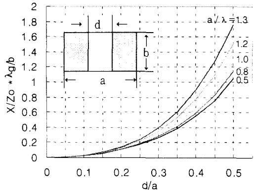
그림 7. T형 등가회로 매개변수와 대칭적 유도성 아이리스의 개구 간격 d의 관계
