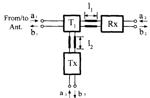
그림 9. 자계면 T-접합을 이용한 다이플렉서 Fig. 9. Diplexer using H-plane T-junction.
