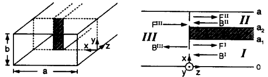
그림 2. 구형 도파관내 E-면 금속삽입에 의한 불연속 구조
