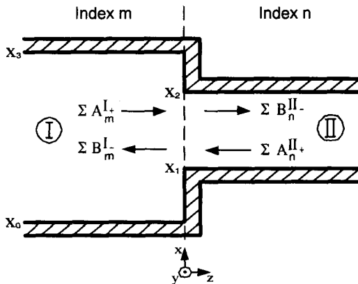
그림 1. 구형 도파관내 대칭적인 자계면 불연속 구조 Fig. 1. Symmetrical H-plane discontinuity in rectangular waveguide.
