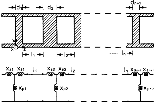
그림 5. 도파관 E-면 금속삽입 구조를 이용한 대역통과 여파기
