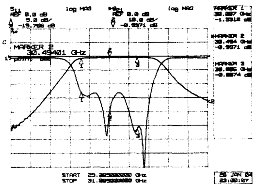
그림 13. 송신 필터의 전달특성 Fig. 13. Transmission characteristics of Tx filter.
