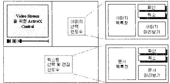
그림 7. 공간동기화 설정화면
