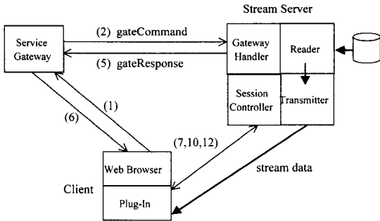
그림 4. 서비스 시나리오
