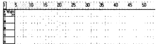
그림 8. 시간동기화 설정화면
