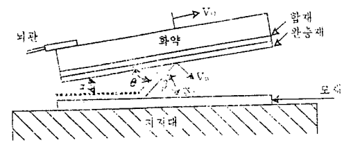
V_1 : 충돌속도 (= 압접속도 : V_1 ), \alpha : 충돌각(동적 경사각)
