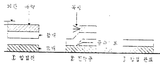
· 금속제트 형성과 압접 과정
