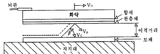
V_c : 충돌속도(=압접속도 : V_w ), \beta : 충돌각(동적 경사각)
