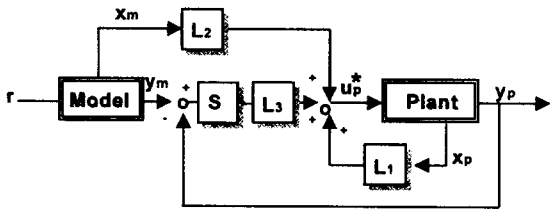
그림 1 강인한 모델추종형 서보시스템의 구성 Fig. 1 Structure of robust model following servo system
