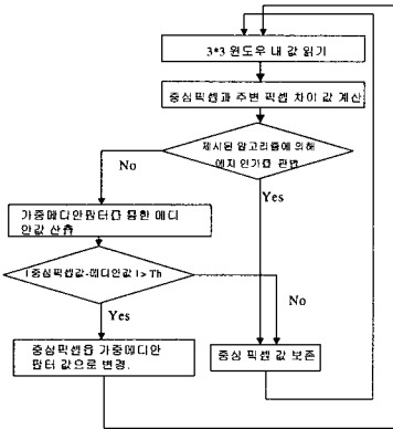
(그림 4) 제시된 알고리즘의 흐름도.
