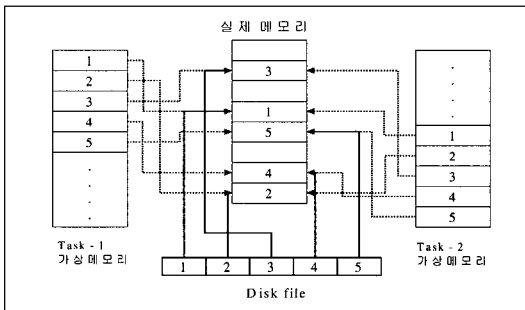
(그림 3) Memory-mapped File 방식에 의한 공유 메모리 설정
