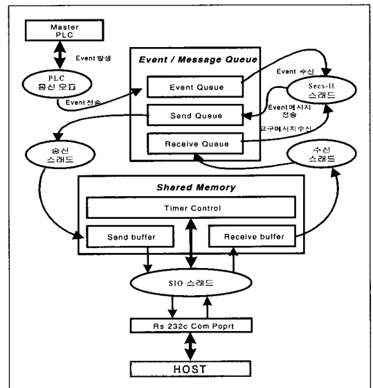
(그림 12) 호스트 통신 모듈의 구조
