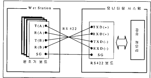
(그림 9) 온도조기와 RS-422 보드간의 통신 구성도
