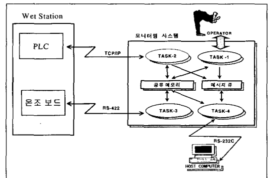
(그림 2) 모니터링 시스템의 구조
