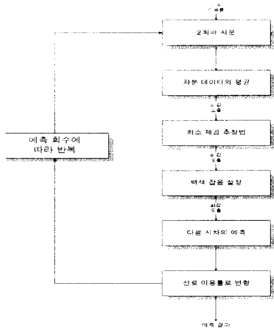
(그림 4) 예측 기법의 전체 알고리즘
