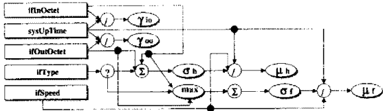
(그림 2) 회선 이용률 분석 계산 모델
