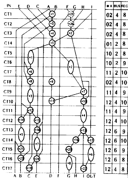
(그림 3) 5차 디지털 웨이브 필터의 DFG 모델
