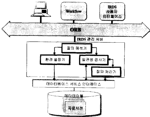
(그림 1) 분산 객체 환경에서의 정보저장소 구조
