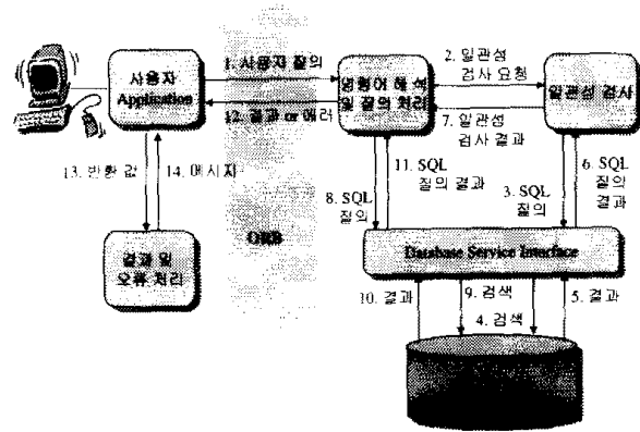
(그림 3) 서비스 수행 절차
