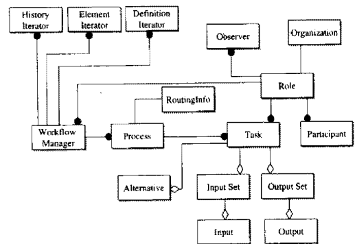
(그림 5) 워크플로우를 위한 IRD 단계의 메타 모델
