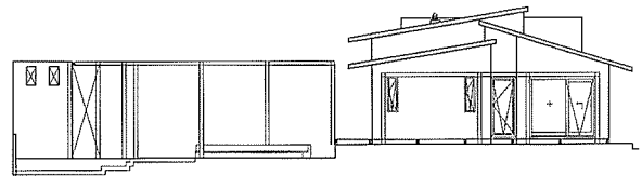
동측면도
