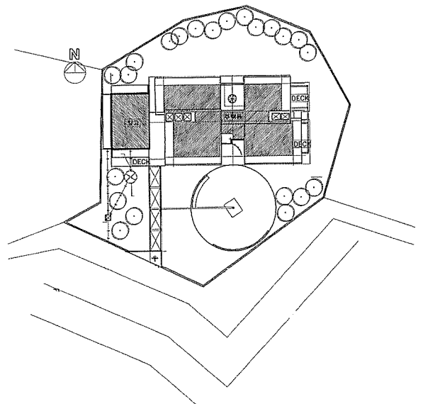
배치도
