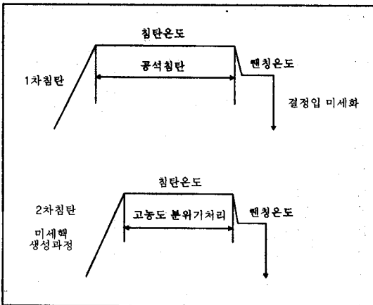
그림 4. Naitoh의 고탄소 침탄 사이클
