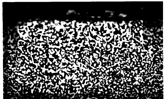
그림 1. 고농도 침탄조직(백색부위 : 탄화물, 흑색부위 : 마르텐사이트 기지)
