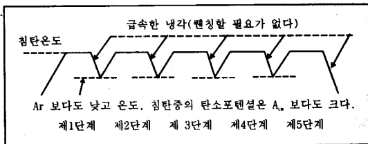
그림 3. O.E. Cullen의 고탄소 침탄 싸이클
