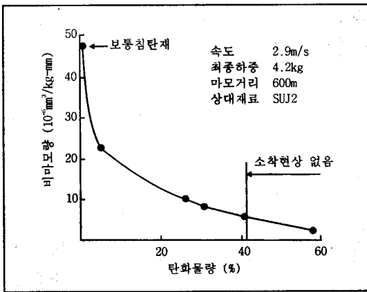
그림 7. 탄화물량과 비마모량
