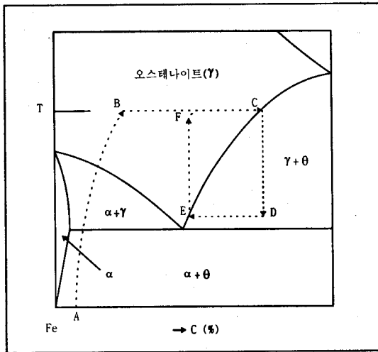
그림 2. 탄화물 생성기구 설명도
