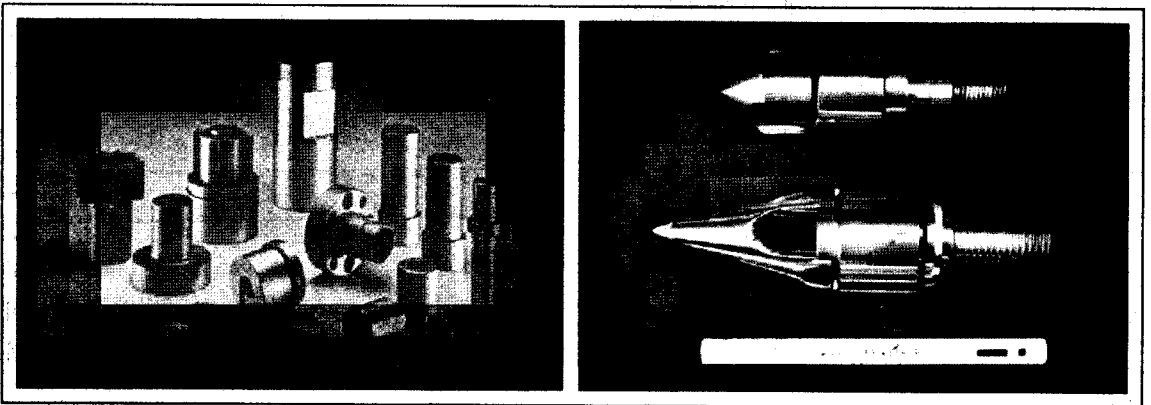
그림 8. 고농도 침탄된 냉간금형(좌)과 플라스틱 사출기 스크류 헤드(우)
