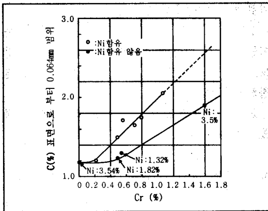
그림 5. Cr과 표면탄소량의 관계
