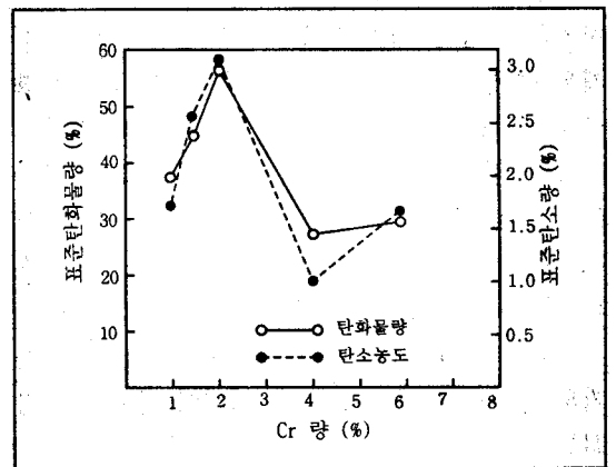
그림 6. Cr량과 탄화물 석출량의 관계
