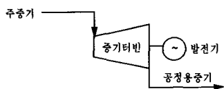
<그림 2> 열병합발전 개념도
