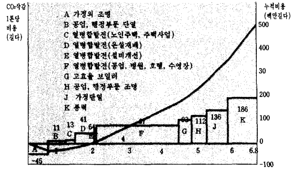
(그림 5) CO 2 삭감수단별 비용대 효과
