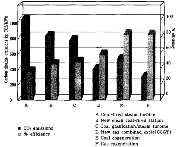
(그림 6) 발전수단별 CO 2 배출량 및 효율 비교
