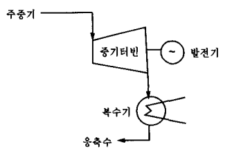
<그림 1> 일반화력발전 개념도
