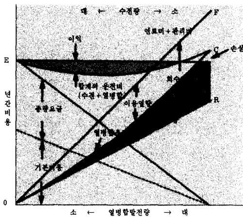
〈그림 4〉 최적발전량 선정예시
