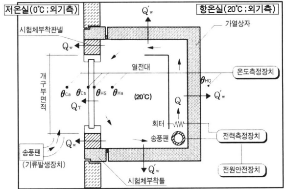
그림 1 시험장치 개요도
