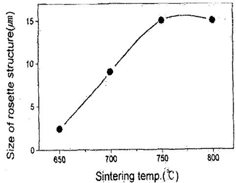
그림 3. 소성온도에 따른 2/65/35 PLZT 박막의 rosette 구조의 크기
