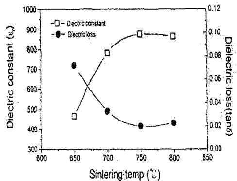
그림 4. 2/65/35 PLZT 박막의 소성온도에 따른 유전상수와 유전손실의 변화
