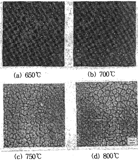
그림 2. 2/65/35 PLZT 박막의 소성온도에 따른 미세구조의 변화
