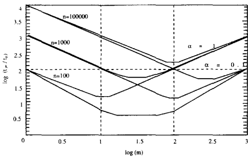
(그림 4) n 와 \alpha 에 대한 부제어국수(m) 폴링 처리시간 (Fig. 4) Polling processing time of m:a for sub control station
