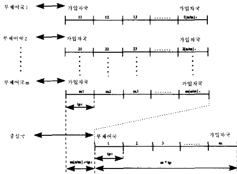
(b) 계층화 구성(b)의 폴링 순서
