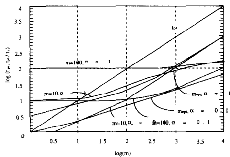
(그림 3) m 와 \alpha 에 대한 사용자국수(n) 폴링 처리시간 (Fig. 3) Polling processing time of m:a for user station
