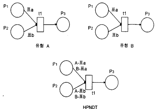
(그림 4) 유형 A에 대한 PNDT와 유형 B에 대한 PNDT를 포개어 HPNDT를 만든 예.
