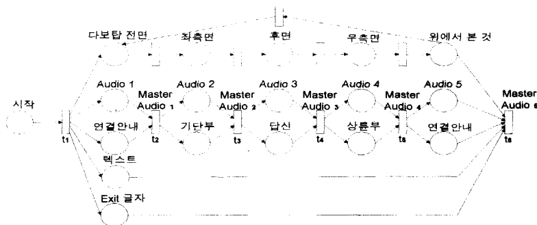
(그림 3) 다보탑 시나리오 중 첫 번째 화면 구성 정보의 페트리넷 모델. (Fig. 3) A Petri net model of the first screen information of the Da-Bo Pagoda scenario.
