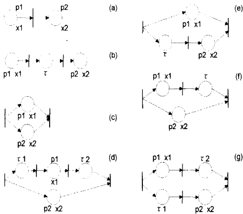
(그림 5) OCPN에 사용된 동기화를 위한 기본 구조. (Fig. 5) Basic OCPN structures for modeling synchronization strategies.
