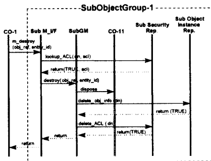
그림 8. 서브객체그룹내에 연산객체 삭제에 대한 ETD Fig. 8. ETD for deletion of object in SubObject Group
