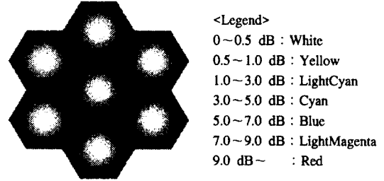
그림 3. 소프트핸드오프 이득의 영역 Fig. 3 Region of soft handoff gain
