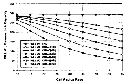
그림 10. 무선가입자망 2의 신호 전력 대 간섭 전력비에 따른 무선가입자망 1의 역방향 링크 용량 (일반화된 거리 = 0.4, 무선가입자망 2의 사용자 수 = 32)
