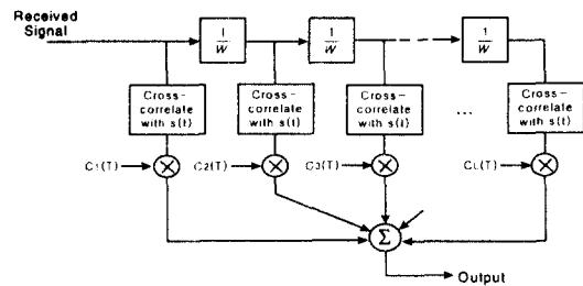
그림 2. RAKE 수신기의 블록 다이어그램 Fig. 2 Block diagram of RAKE receiver.
