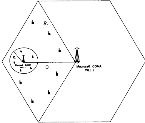
그림 3. 중첩된 매크로셀과 마이크로셀 W-CDMA 무선가입자망의 구조
