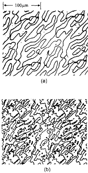
그림 4. 광 리소그래피로 제작된 위상홀로그래프의 현미경사진. (a) 위상차가 \pi 인 주 홀로그래프, (b) 위상차가 \pi/2 인 보조 홀로그래프. Fig 4. The microscopic picture of the fabricated phase holograms. (a) Main hologram of phase \pi , (b) Subhologram of phase \pi/2
