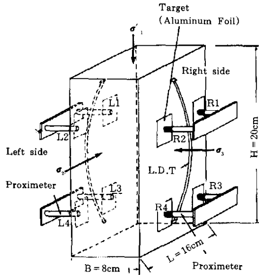
그림 3. 미소 변형 측정장치
