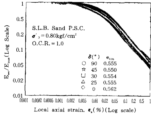
그림 27. \delta 에 대한 E_{sec}/E_{max} 과 \epsilon_1 과의 관계 (정규압밀 SLB 모래)
