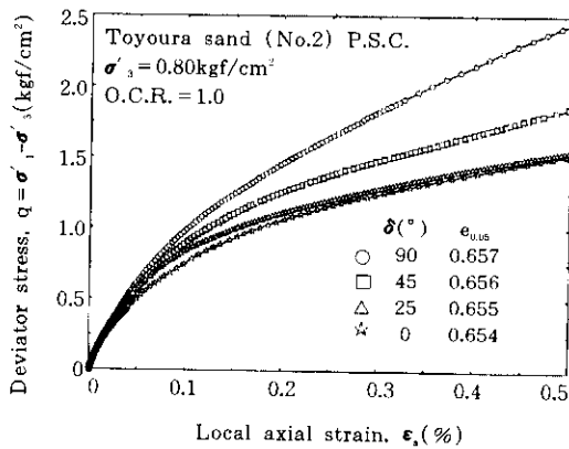
그림 5. \epsilon_1 = 0.5\% 까지의 응력-변형률 관계 (정규압밀 Toyoura 모래)
