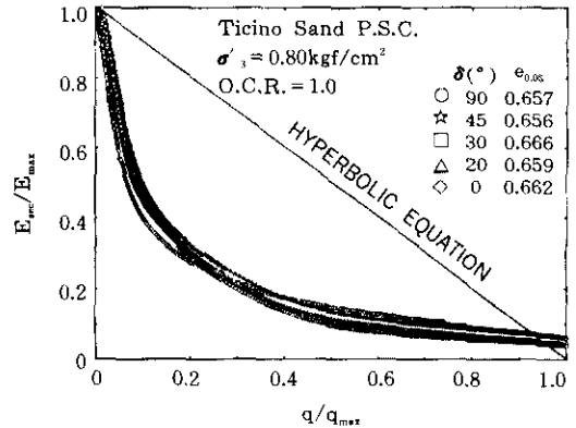
그림 35. E_{sec}/E_{max} \sim q/q_{max} 의 관계 (정규압밀 Ticino 모래)
