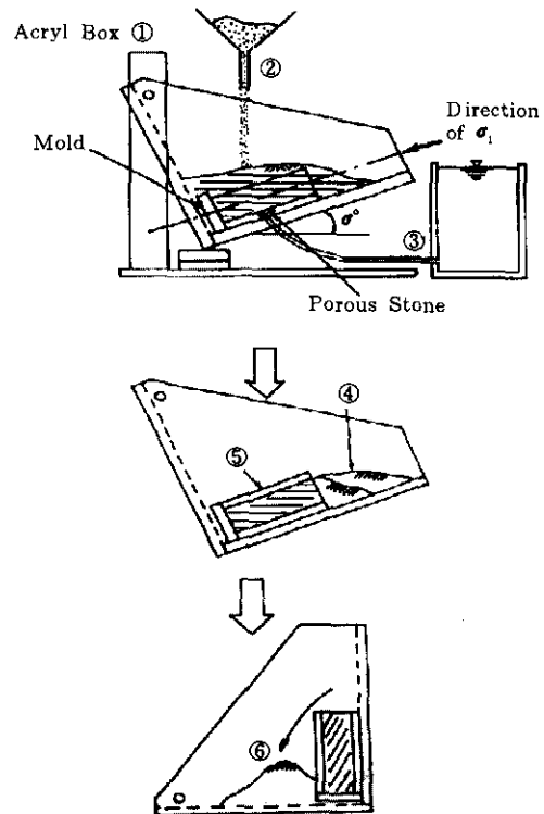
그림 4. \delta 공시체의 제작과정
