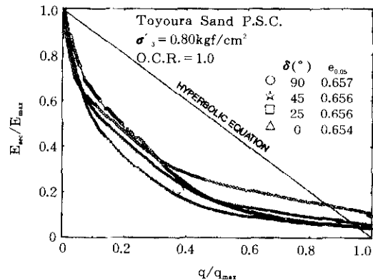
그림 31. E_{sec}/E_{max} \sim q/q_{max} 의 관계 (정규압밀 Toyoura 모래)
