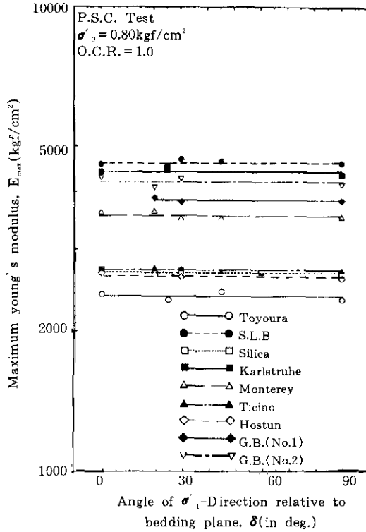
그림 23. \delta 에 대한 E_{max} (각 정규압밀공시체)
