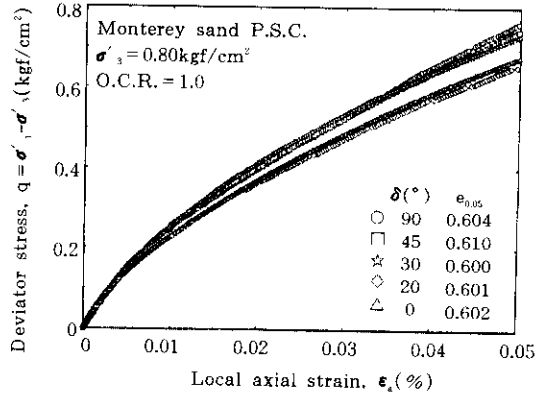
그림 13. \epsilon_1 = 0.05\% 까지의 응력-변형률 관계 (정규압밀 Monterey 모래)
