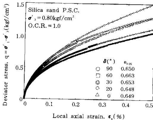
그림 7. \epsilon_1 = 0.5\% 까지의 응력-변형률 관계 (정규압밀 Silica 모래)
