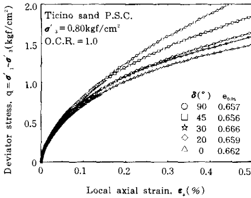
그림 9. \epsilon_1 = 0.05\% 까지의 응력-변형률 관계 (정규압밀 Ticino 모래)
