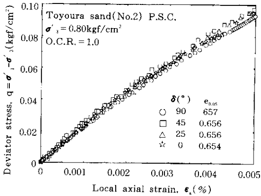
그림 15. \epsilon_1 = 0.005\% 까지의 응력-변형률 관계 (정규압밀 Toyoura 모래)
