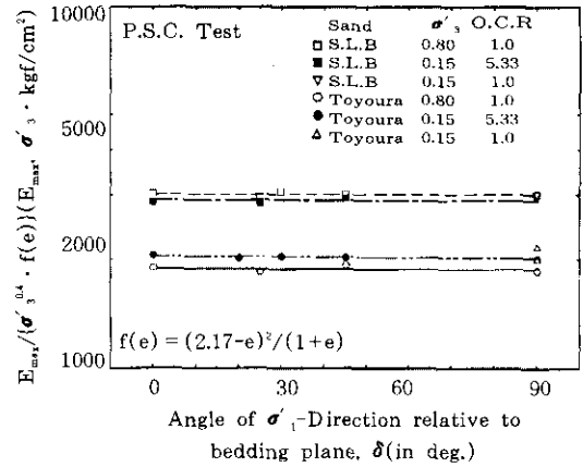
그림 24. 정규화한 E_{max} 과 \delta 와의 관계(Toyoura모래와 SLB모래의 정규압밀·과압밀공시체)
