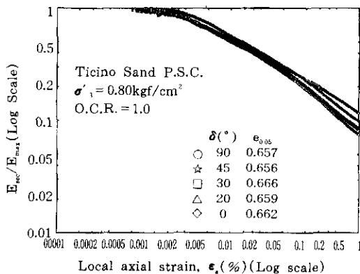
그림 30. \delta 에 대한 E_{sec}/E_{max} 과 \epsilon_1 과의 관계 (정규압밀 Ticino 모래)
