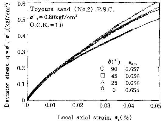
그림 10. \epsilon_1 = 0.05\% 까지의 응력-변형률 관계 (정규압밀 Toyoura 모래)
