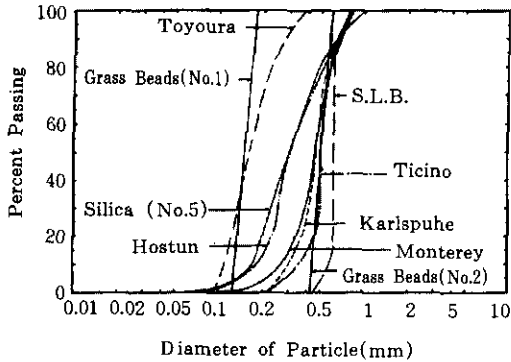
그림 1. 각 시료의 입경가적곡선
