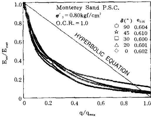
그림 34. E_{sec}/E_{max} \sim q/q_{max} 의 관계 (정규압밀 Monterey 모래)
