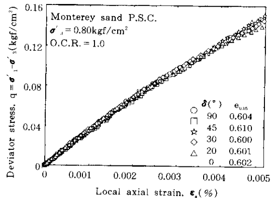
그림 18. \epsilon_1 = 0.005\% 까지의 응력-변형률 관계 (정규압밀 Monterey 모래)
