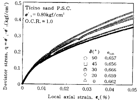
그림 14. \epsilon_1 = 0.05\% 까지의 응력-변형률 관계 (정규압밀 Ticino 모래)
