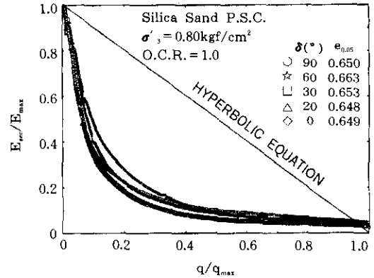
그림 33. E_{sec}/E_{max} \sim q/q_{max} 의 관계 (정규압밀 Silica 모래)
