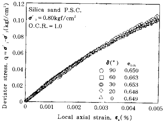
그림 17. \epsilon_1 = 0.005\% 까지의 응력-변형률 관계 (정규압밀 Silica 모래)
