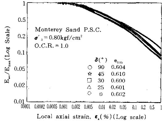
그림 29. \delta 에 대한 E_{sec}/E_{max} 과 \epsilon_1 과의 관계 (정규압밀 Monterey 모래)
