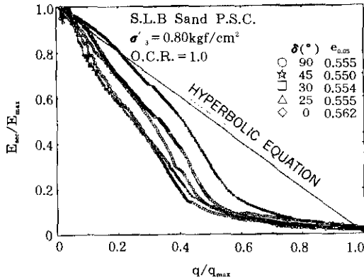
그림 32. E_{sec}/E_{max} \sim q/q_{max} 의 관계 (정규압밀 SLB 모래)
