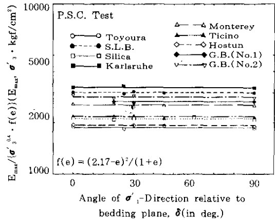
그림 25. 정규화한 E_{max} 과 \delta 와의 관계(각 정규압밀공시체)
