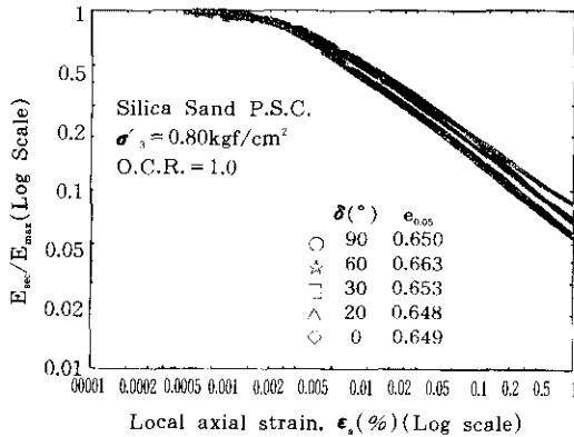
그림 28. \delta 에 대한 E_{sec}/E_{max} 과 \epsilon_1 과의 관계 (정규압밀 Silica 모래)
