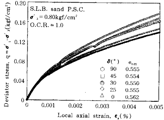
그림 16. \epsilon_1 = 0.005\% 까지의 응력-변형률 관계 (정규압밀 SLB 모래)
