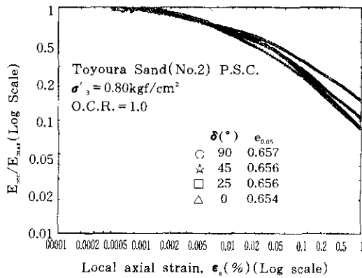
그림 26. \delta 에 대한 E_{sec}/E_{max} 과 \epsilon_1 과의 관계 (정규압밀 Toyoura 모래)
