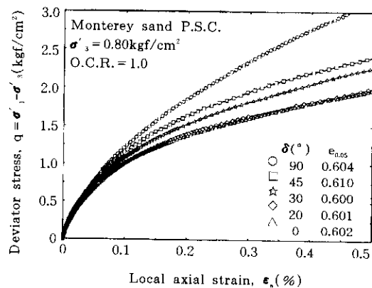
그림 8. \epsilon_1 = 0.5\% 까지의 응력-변형률 관계 (정규압밀 Monterey 모래)
