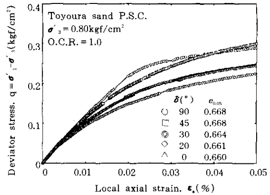
그림 20. \epsilon_1 = 0.05\% 까지의 응력-변형률 관계 (과압밀 Toyoura 모래)
