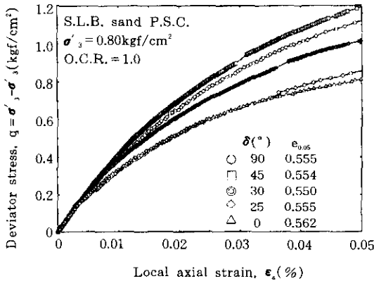
그림 11. \epsilon_1 = 0.05\% 까지의 응력-변형률 관계 (정규압밀 SLB 모래)
