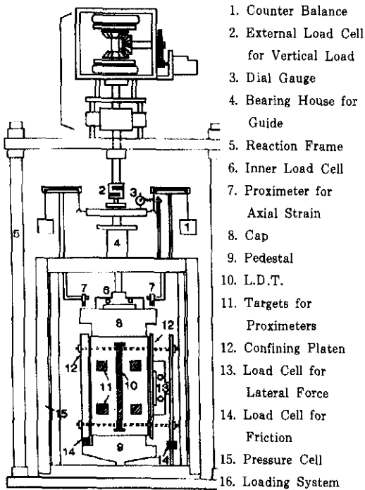
그림 2. 실험장치의 개략도
