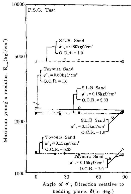
그림 22. \delta 에 대한 E_{max} (Toyouira 모래와 SLB 모래의 정규압밀·과압밀공시체)
