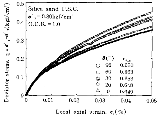
그림 12. \epsilon_1 = 0.05\% 까지의 응력-변형률 관계 (정규압밀 Silica 모래)
