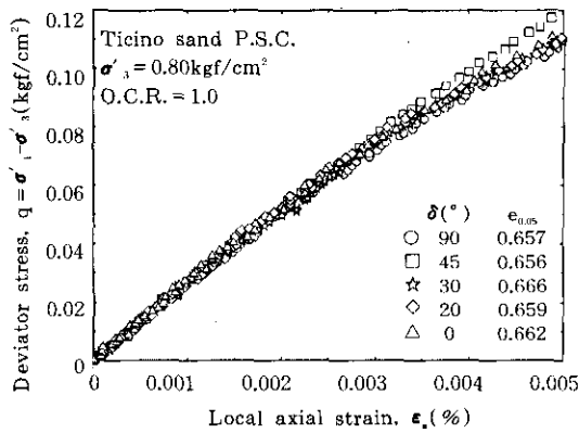
그림 19. \epsilon_1 = 0.005\% 까지의 응력-변형률 관계 (정규압밀 Ticino 모래)
