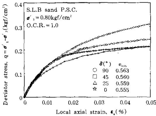
그림 21. \epsilon_1 = 0.05\% 까지의 응력-변형률 관계 (과압밀 SLB 모래)
