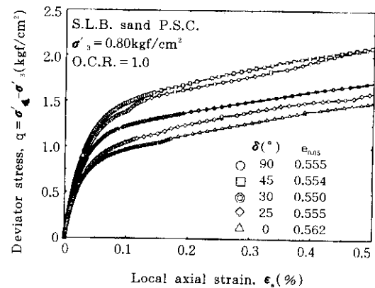
그림 6. \epsilon_1 = 0.5\% 까지의 응력-변형률 관계 (정규압밀 SLB 모래)
