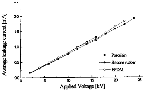
그림 4. 증류수 분무시 각 재료의 평균누설전류의 특성
