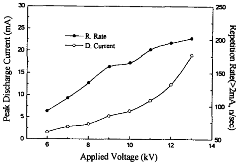
그림 8. porcelain의 건조시 전압에 따른 scintillation 방전 특성
