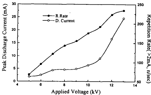
그림 9. porcelain의 0.5 wt% NaCl 분무후 30분 경과시 scintillation 방전 특성
