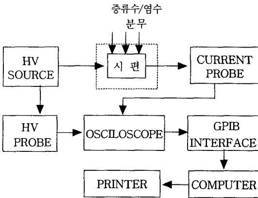
그림 2. 실험장치의 블록도
