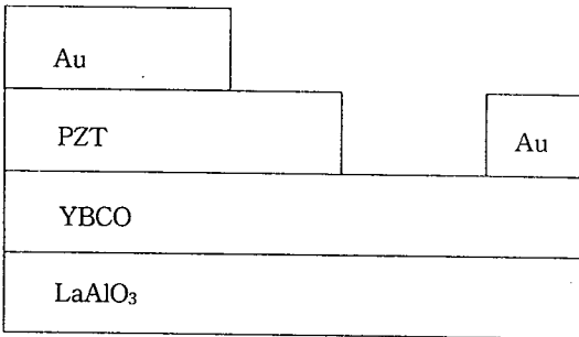
그림 2. Au/PZT/YBCO/LaAlO 3 박막의 구조 Fig. 2. Au/PZT/YBCO/LaAlO 3 heterostructure
