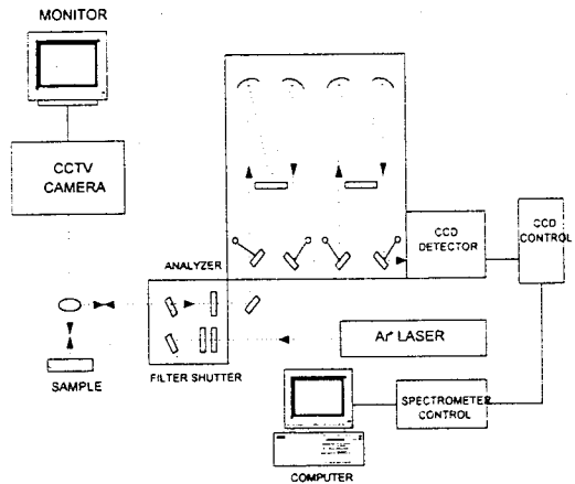
그림 1. 마이크로 라만 분광기기
