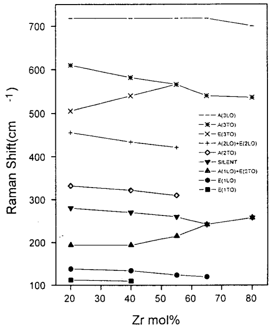
그림 5. Zr 몰비에 따른 각 진동 모드의 변화 Fig. 5. Variation of each vibration mode for Zr mol %
