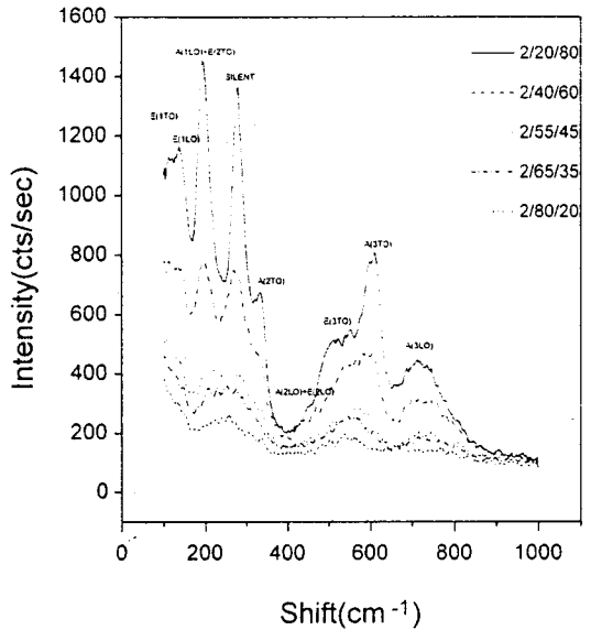
그림 4. Zr/Ti 조성비에 따른 PLZT 박막의 라만 스펙트라
