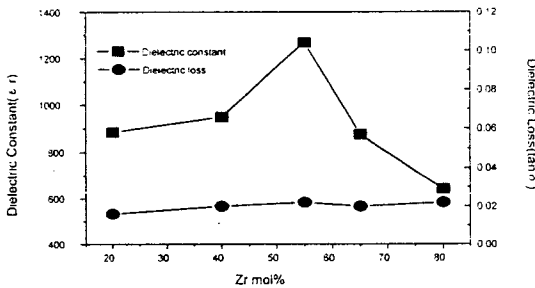
그림 6. Zr/Ti비에 따른 PLZT 박막의 유전상수와 유전손실의 변화 Fig. 6. Variation of dielectric constant and loss of PLZT thin film with Zr/Ti ratios
