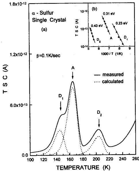
그림 4.(a) \alpha -sulfur 단결정의 TSC 스펙트럼.
