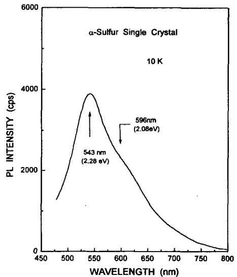
그림 3. \alpha -sulfur 단결정의 광발광 스펙트럼. Fig. 3. Photoluminescence spectrum of \alpha -sulfur single crystal
