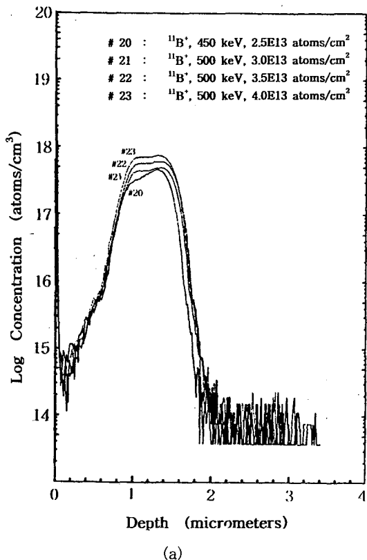
그림 2. 1000°C, 15초, 질소분위기 급속열처리후의 붕소 농도분포. (a) 주입량 변화. (b) 에너지 변화. Fig. 2. Boron concentration profiles after 1000°C, 15sec., N 2 ambient Rapid Thermal Annealing. (a) dose variation. (b) energy variation.
