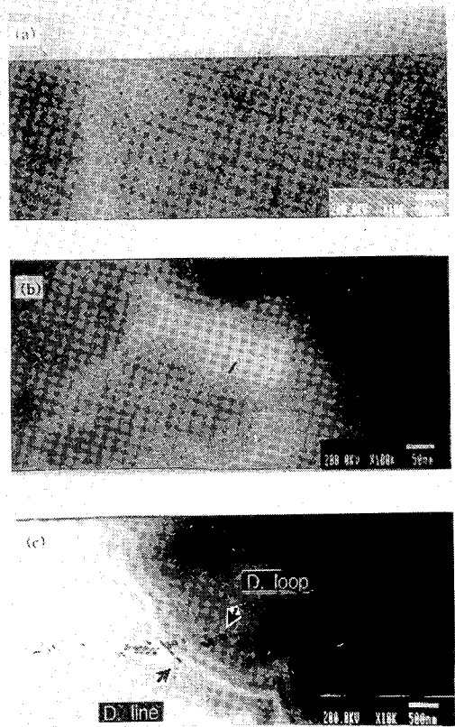
그림 4. 950°C, 30분, 질소분위기 열처리후 투과전자현미경에 나타난 2차결함. (a) 1MeV, 31 P + , 3E13/cm 2 . (b) 1MeV, 31 P + , 1E14/cm 2 . (c) 1MeV, 31 P + , 3E14/cm 2 .
