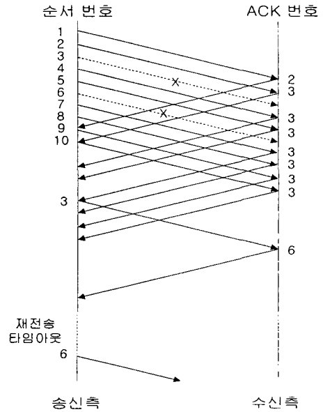
그림 3. 고속 재전송 알고리즘을 사용하는 경우에 재전송 타임아웃이 유발되는 과정 Fig. 3. An example of timeout for fast retransmit algorithm
