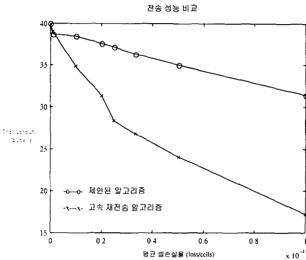
그림 7. 40Mbps 대역폭으로 전송하는 경우의 셀 손실에 따른 성능 변화 Fig. 7. Performance comparison for 40Mbps bandwidth channel
