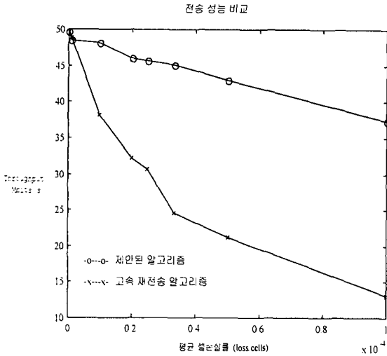
그림 6. 50Mbps 대역폭으로 전송하는 경우의 셀 손실에 따른 성능 변화 Fig. 6. Performance comparison for 50Mbps bandwidth channel
