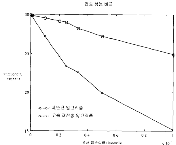
그림 8. 30Mbps 대역폭으로 전송하는 경우의 셀 손실에 따른 성능 변화 Fig. 8. Performance comparison for 30Mbps bandwidth channel
