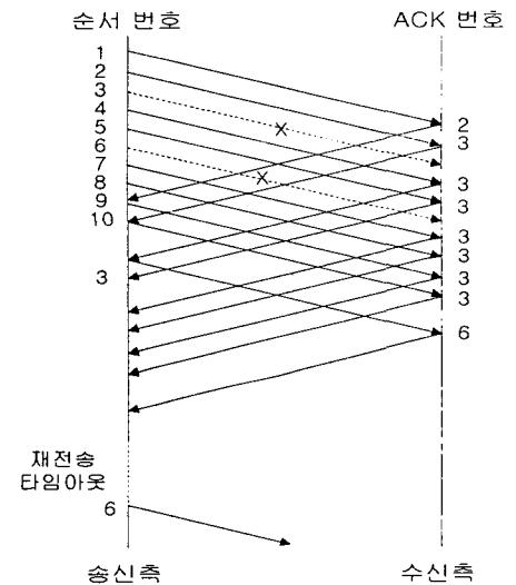
그림 4. 슈퍼 고속 재전송 알고리즘을 사용하는 경우에 재전송 타임아웃이 유발되는 과정 Fig. 4. An example of timeout for super fast retransmit algorithm
