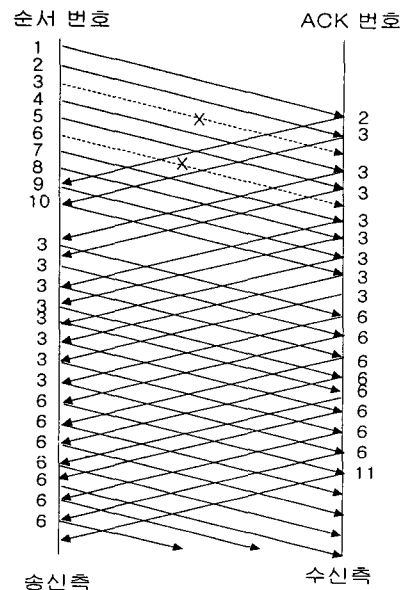
그림 5. 재전송 타임 아웃이 제거된 과정 Fig. 5. An example of timeout removal
