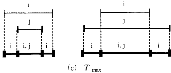
(그림 1) T_{min} , T_{mia} , T_{max} 의 고정 간격 집합 (Fig. 1) Constant Interval Sets for T_{min} , T_{mia} , T_{max}
