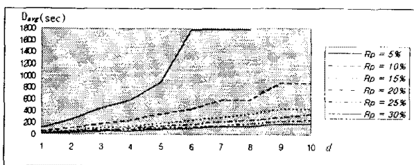
(b) k=6
