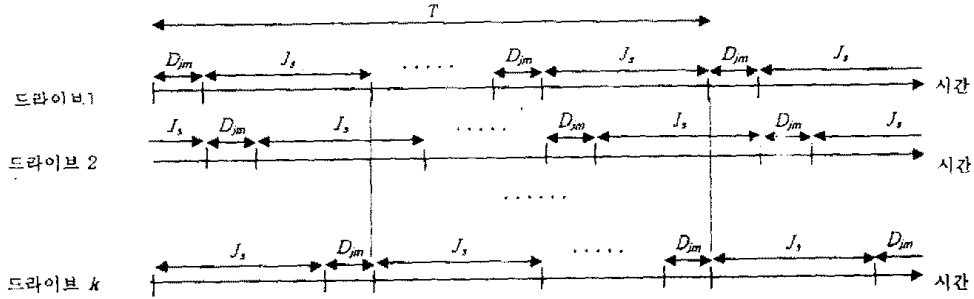
(그림 2) 광자기 디스크 교환 시간을 은폐시키는 스케줄링 방법 (Fig. 2) A scheduling method to hide the optical disk swapping time
