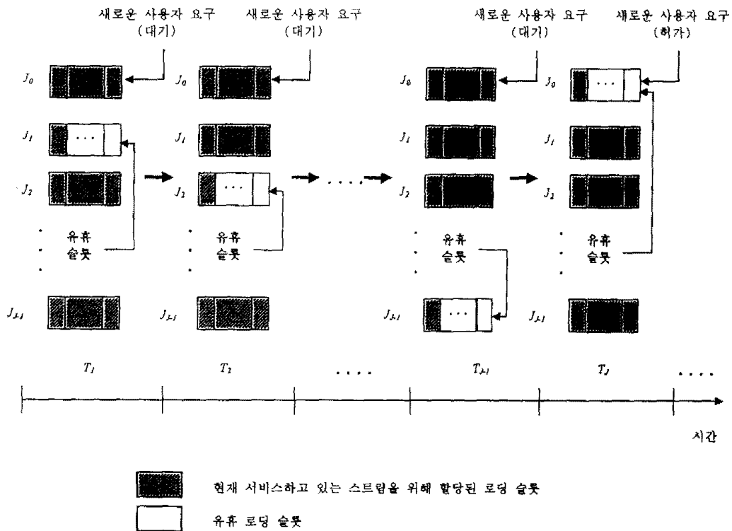
(그림 6) 분산 저장 방법과 로딩 슬롯 (Fig. 6) Loading slots in distributed allocation method
