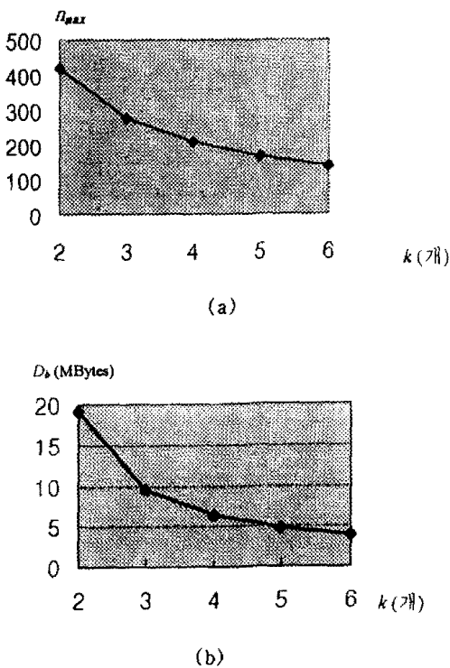
(그림 7) 시스템 변수간의 연관 관계 (Fig. 7) Relationship among system parameters
