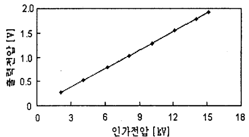
그림 9. 교류인가전압과 전압측정장치의 출력전압 관계 Fig. 9. Relation between output voltage of the voltage measuring device and AC applied voltages
