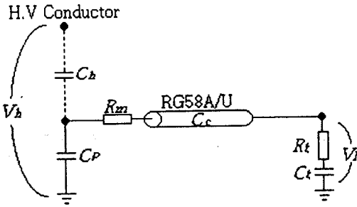
그림 3. 전압측정회로의 기본 구성 Fig. 3. Basic construction of a voltage measuring circuit
