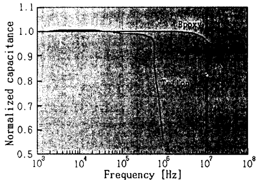
그림 4. 검출전극용 절연재료의 주파수 특성 Fig. 4. Frequency characteristics of insulation materials for the detecting electrode
