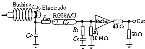
그림 5. 전압측정장치의 구성 Fig. 5. Construction of the voltage measuring device
