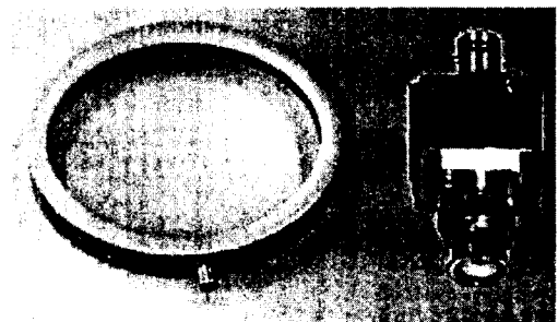
그림 2. 검출전극과 접속장치의 구조 Fig. 2. Construction of the detecting electrode and the connector
