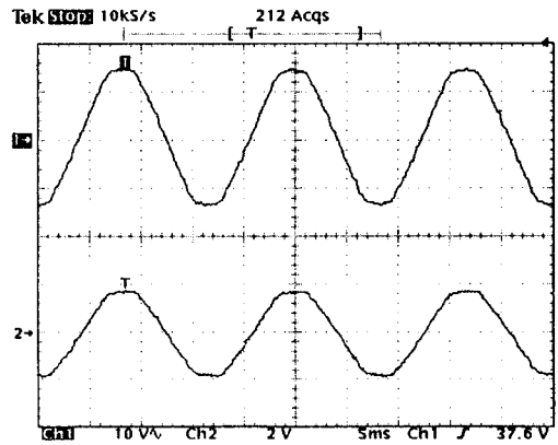
상: 입력전압파형(고전압프로브) 하: 응답파형(전압측정장치) 그림 8. 상용주파수 전압에서 전압측정장치의 응답파형 예
