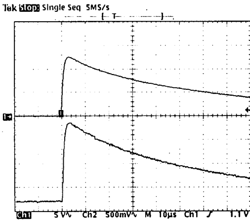
상: 입력전압파형(고전압프로브) 하: 응답파형(전압측정장치) 그림 10. 비진동성 충격전압에 대한 전압측정장치의 응답파형
