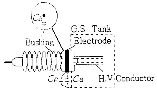
그림 1. 가스절연개폐기에서 전압측정원리 Fig. 1. Principle of voltage measuring in a gas-filled switch.
