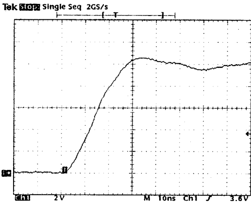
그림 7. 직각과 입력에 대한 전압측정장치 응답파형 Fig. 7. Response waveform of the voltage measuring device to a step pulse input
