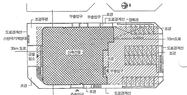
배치도
