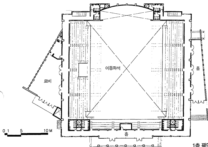
1층 평면도
