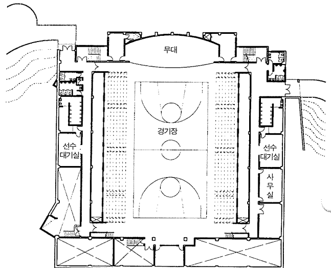
지하층 평면도
