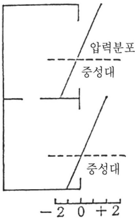
(a) 2층 건물의 1층에서 화재가 발생한 경우 중성대가 2개 생성하는 예
