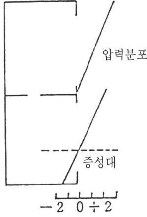
(b) 2층 건물의 1층에서 화재가 발생한 경우 중성대가 2개 생성하는 예
