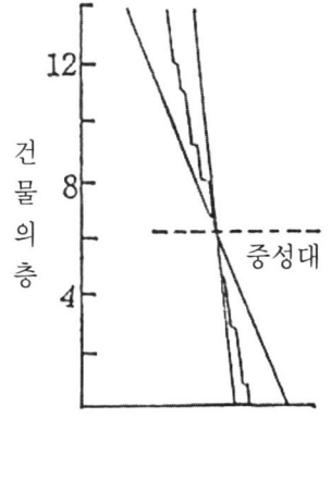
(c) 난방중인 경우에 고층빌딩(14층)의 압력분포와 중성대
