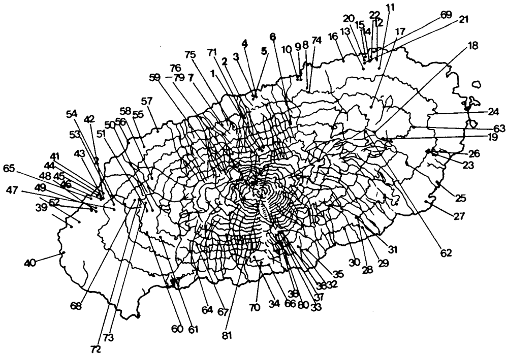
그림 2. 제주도의 동굴분포
