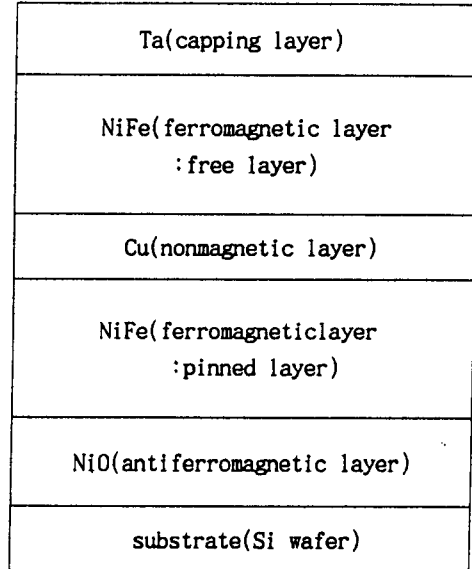
그림 2. 시편의 구조에 대한 모식도
