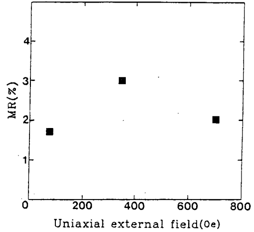
그림 4. 일축자기장 변화에 따른 Si/SiO 2 /NiO(420Å)/NiFe(50Å)/Cu(30Å)/NiFe(50Å)/Ta(50Å) 샌드위치의 자기저항비
