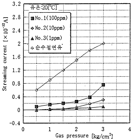
그림 6. 유동전류와 가스압의 관계 Fig. 6. The relationship between streaming current and gas pre.
