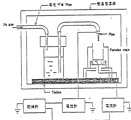
그림 1. 실험장치 구성도
