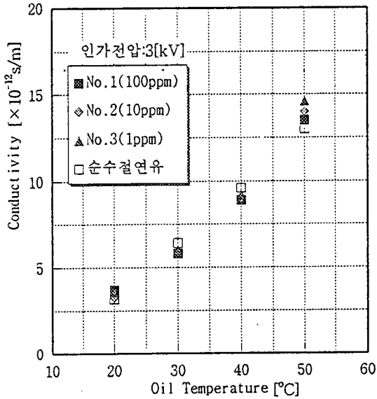
그림 9. 도전율과 유온의 관계
