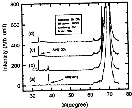
그림 1. 기판온도에 대한 X선 회절도의 변화 (a) 상온 (b) 100°C (c) 200°C (d) 300°C
