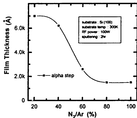
그림 7. 질소비율에 대한 증착율의 변화 Fig. 7. Variation of the deposition rate on the N 2 ratio
