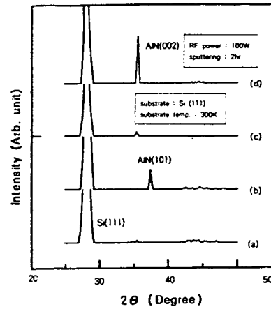
그림 6. 질소비율에 대한 X선 회절도의 변화 (AlN/Si(111)) (a) 20% (b) 40% (c) 80% (d) 100%
