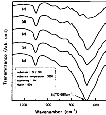
그림 2. 고주파출력에 대한 적외선 분광의 변화 (a) 140W (b) 120W (c) 100W (d) 60W (e) 40W
