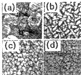
사진 1. 질소비율에 대한 표면의 변화: (기판: Si (100), 기판온도: 300K, 고주파 출력: 100W, 때려내기 시간 : 1hr) : (a) 20% (b) 40% (c) 80% (d) 100% Photo. 1 Variation of the surface morphology on the N 2 ratio (substrate : Si (100), substrate temperature : 300K, RF power : 100W, sputtering : 1hr ) : (a) 20% (b) 40% (c) 80% (d) 100%
