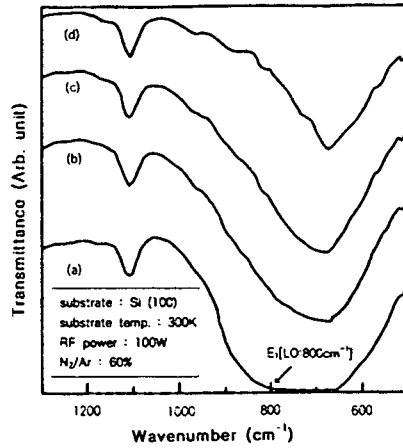
그림 4. 때려내기 시간에 대한 적외선 분광의 변화 : (a) 4hr (b) 3hr (c) 2hr (d) 1hr Fig. 4. Variation of the IR spectrum on the sputtering duration : (a) 4hr (b) 3hr (c) 2hr (d) 1hr
